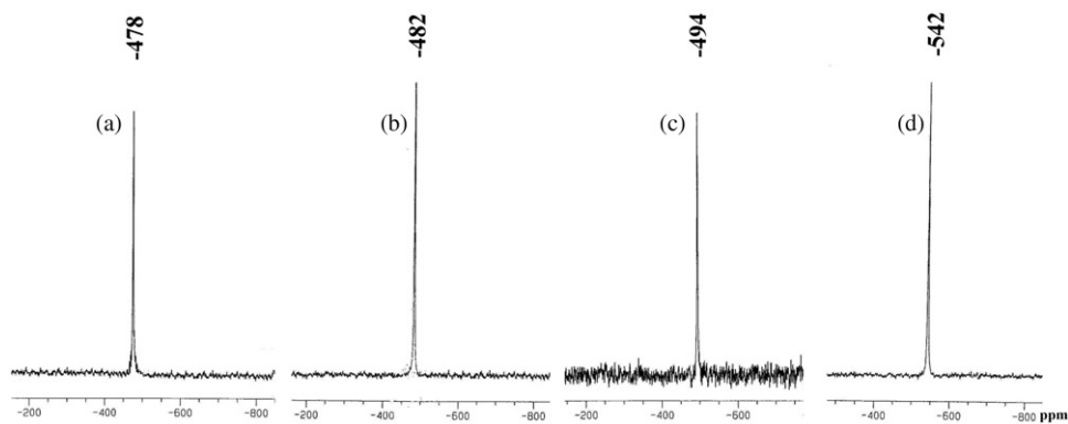
Figure 5. ^{51}\text{V} NMR spectra of (a) 1 , (b) 2 , (c) 3 , and (d) 4 .
